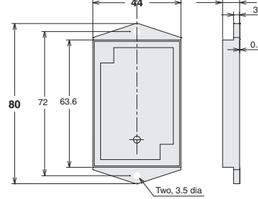
E39-RP1
