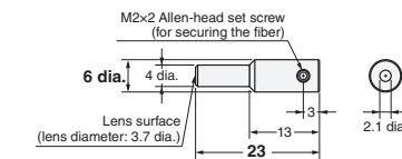
E39-F3A
